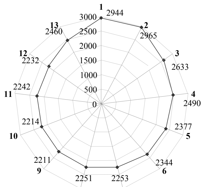
Figura 3. Involuția populației stabile în comună (legendă: 1 – anul 1990, 13 – anul 2002).
